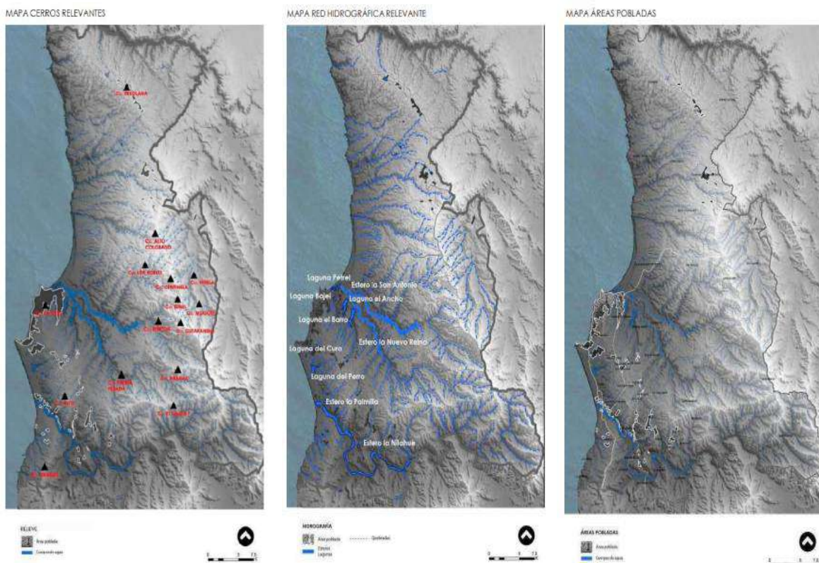
Figura 45: Contexto Geomorfológico.
