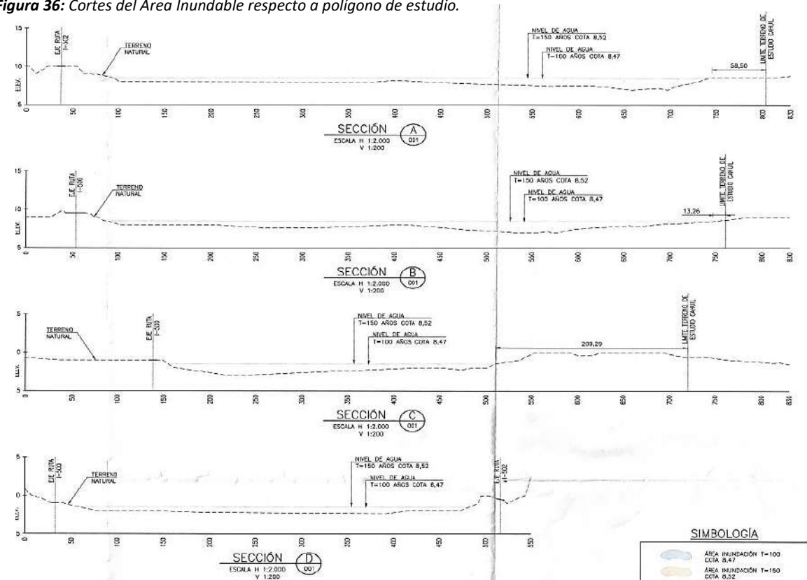
Figura 36: Cortes del Área Inundable respecto a polígono de estudio.
